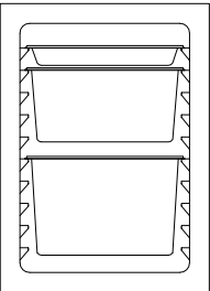
54L 1 x GN 1/1-40 1 x GN 1/1-150 1 x GN 1/1-200
