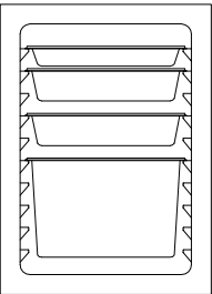
50L 1 x GN 1/1-40 2 x GN 1/1-65 1 x GN 1/1-200
