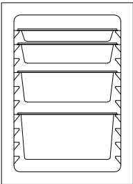
48L 1 x GN 1/1-40 1 x GN 1/1-65 1 x GN 1/1-100 1 x GN 1/1-150
